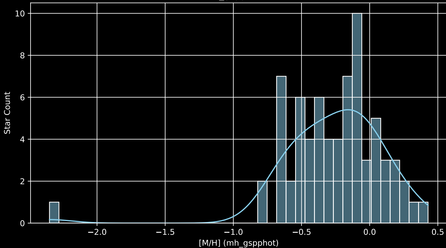
GALAH DR4 Field: [7358] [M/H] (mh_gspphot) (n= 71)
