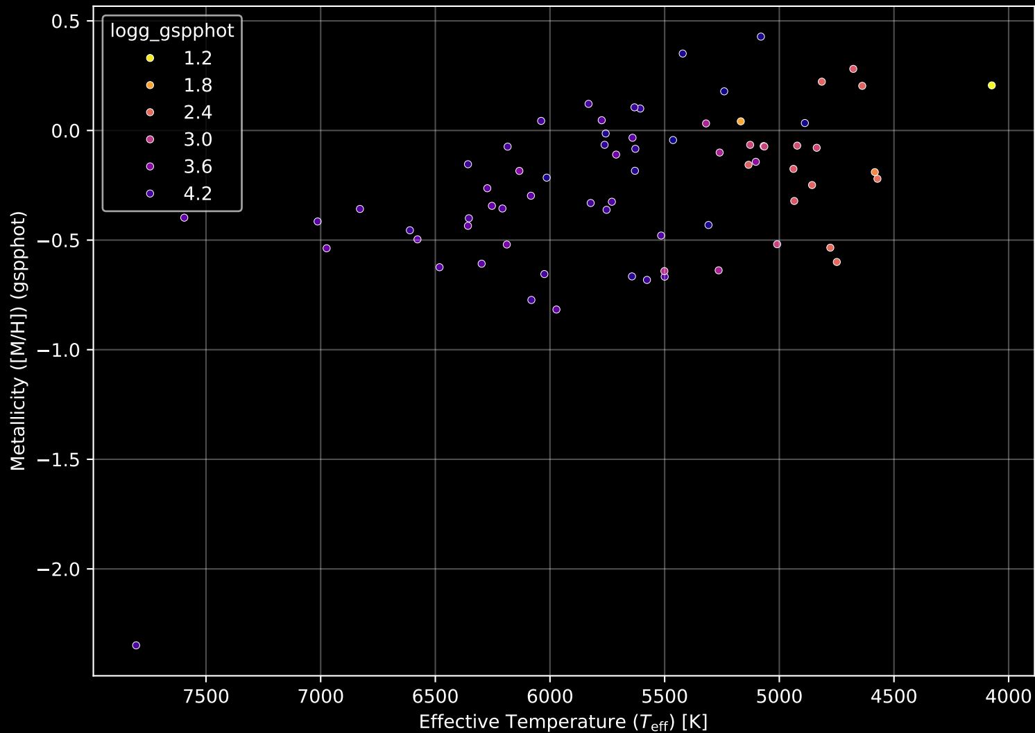
GALAH DR4 Field: [7358] Stellar Population Parameters (n= 71)
