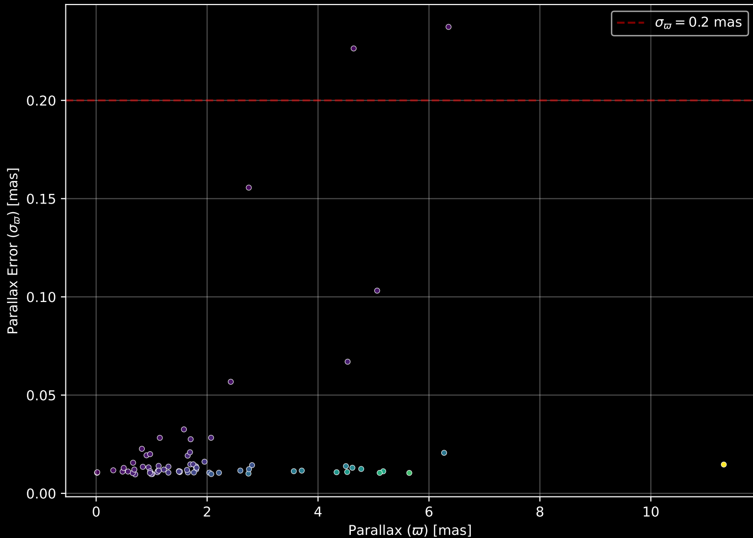
GALAH DR4 Field: [7358] Parallax Quality (n= 71)
