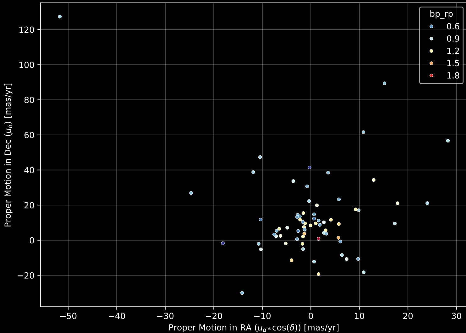
GALAH DR4 Field: [7358] Proper Motion Diagram (n= 71)
